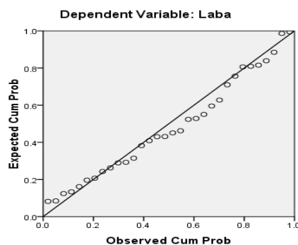
Gambar. 1 Uji normalitas
