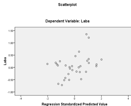
Gambar 2. Uji Heterokedastisitas
